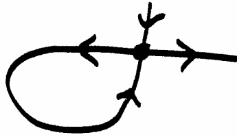
Homoclinic orbits
