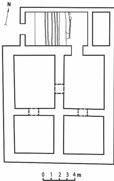
Плян підвального поверху палацу Мазепи на передмісті Батурина Гончарівці (перед 1700 р.) за археологічними дослідями. Реконструкція Ю. Ситого, комп'ютерна графіка С. Дмитрієнка, 2013 р.
